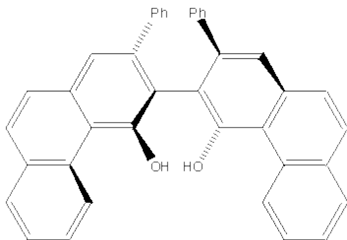
S-VAPOL
