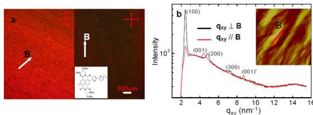
强磁场 (8T) 下生长的P (NDI20D-T2) 薄膜的宏观取向结构: (a) 极化光显微图; (b) In-plane掠入射X光衍射图 (GIXRD)
