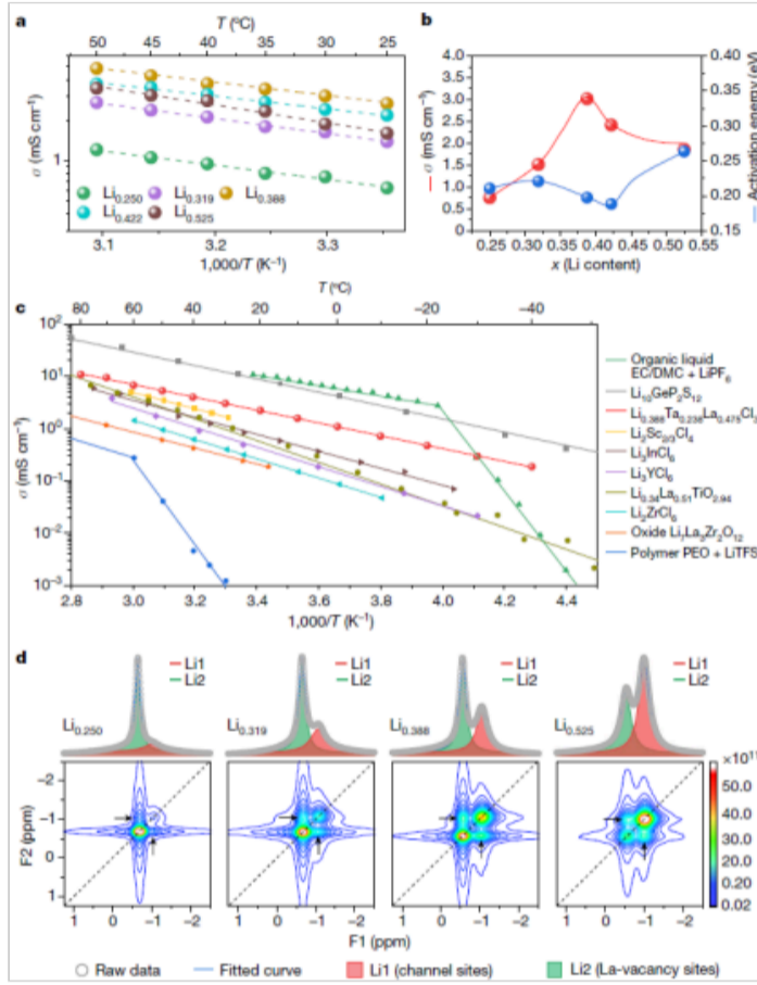
图2. LaCl 3 基固态电解质的离子传输性能和机制
