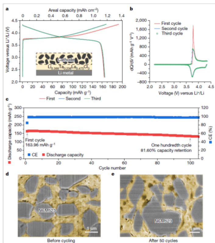
图4.LaCl 3 基固态电解质的全固态锂金属电池
