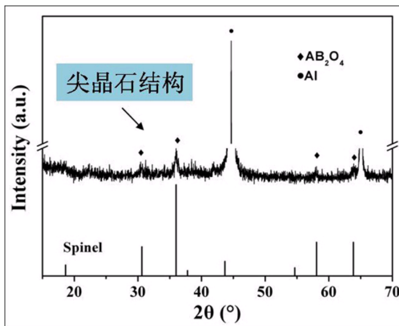
图1 尖晶石型陶瓷吸热涂层的XRD图
