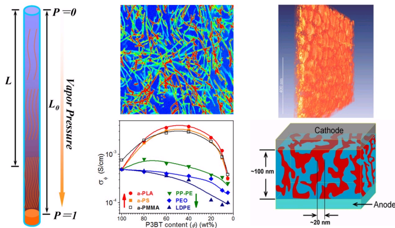
左：可控溶剂气氛处理装置示意图；中：绝缘基质增强的半导体高分子导电率及其形态；右：聚合物太阳能电池光敏薄膜3D形态与模型。
