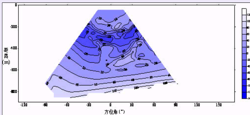
图1 井中瞬变电磁法在煤矿独头巷道超前探测电阻率垂直剖面图
