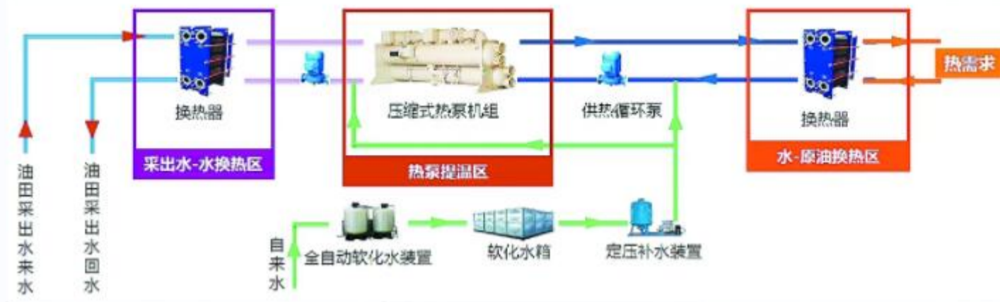
余热+压缩式热泵工艺流程图
