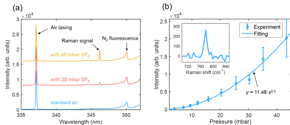
图2 利用空气激光辅助的单光束相干拉曼光谱技术，实验测得的 (a) \text{SF}_6 拉曼信号以及 (b) 拉曼信号强度与气体浓度的定量关系。插图：空气中浓度为0.38%的 \text{SF}_6 气体的拉曼信号。
