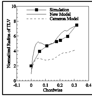
图2 泄漏流作用区域大小的预测结果
