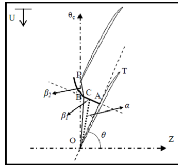
图3 失速临界点交界面位置模型
