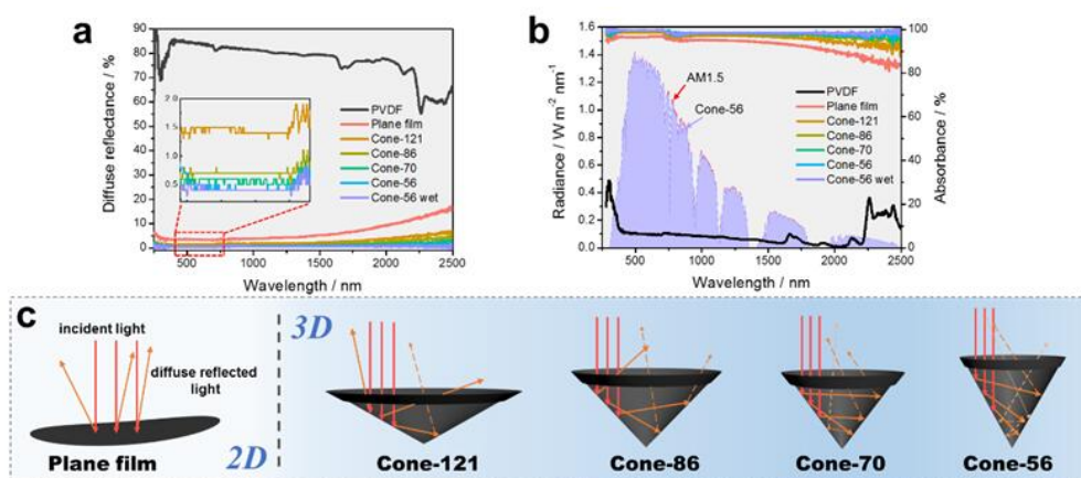
图2. 3D空心锥形膜与2D平面膜样品的漫反射性能对比 (a) 及吸光率对比 (b)，多步反射过程示意图 (c)
