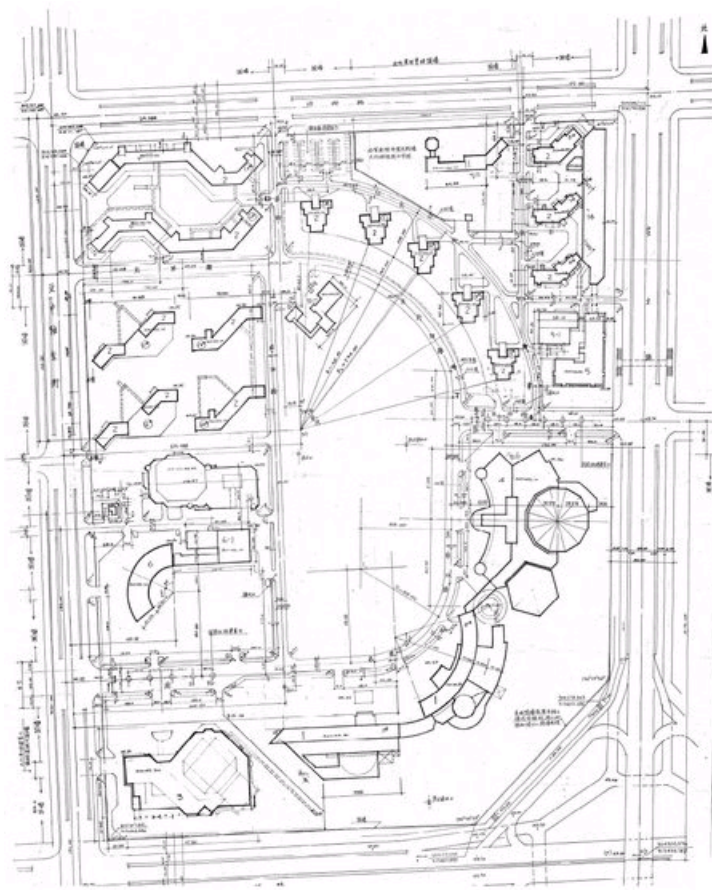
总平面
