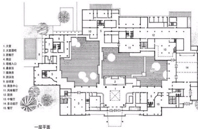
一层平面
