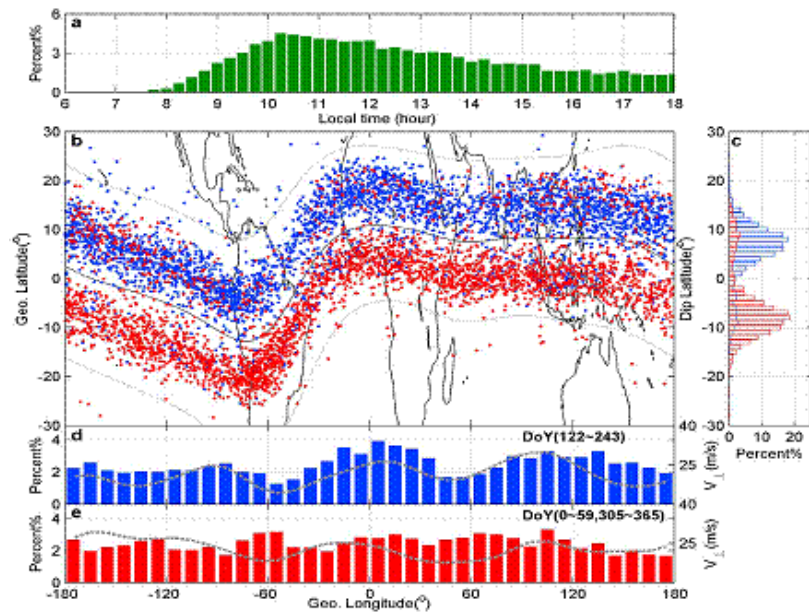
附图说明：电离层分层结构的纬度和经度变化性特征
