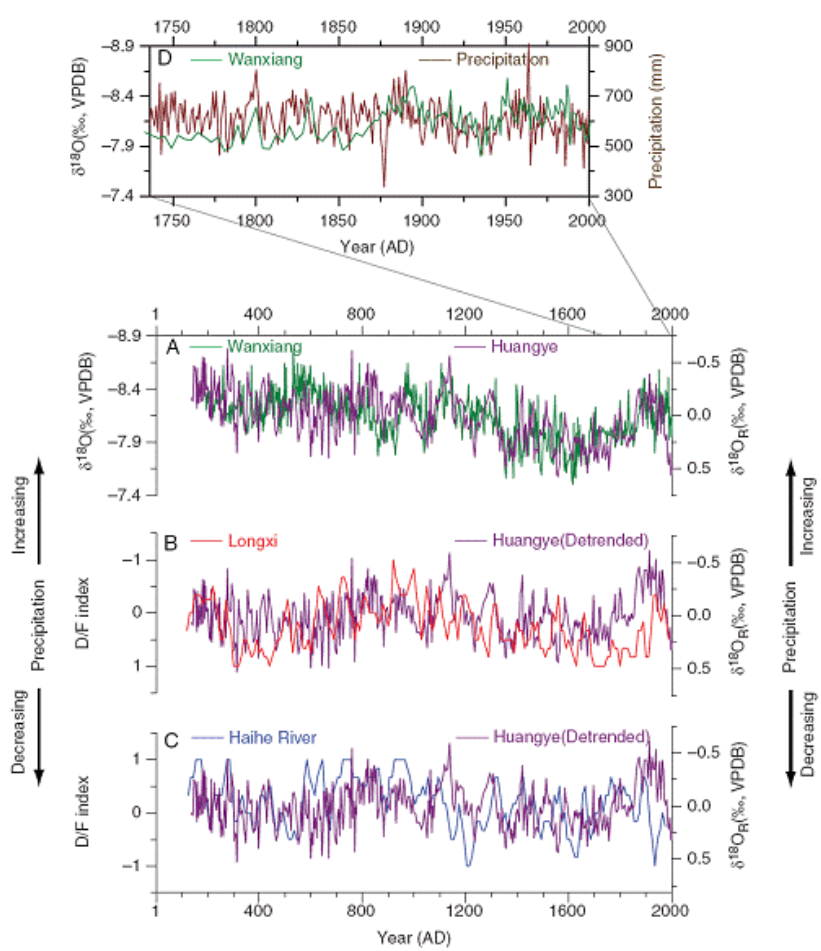
黄谷洞石笋记录和中国北方半湿润区其他降雨记录对比
