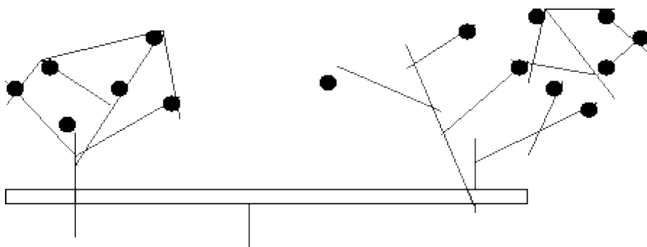
图 7 — 3 星型—网状混合型接地
