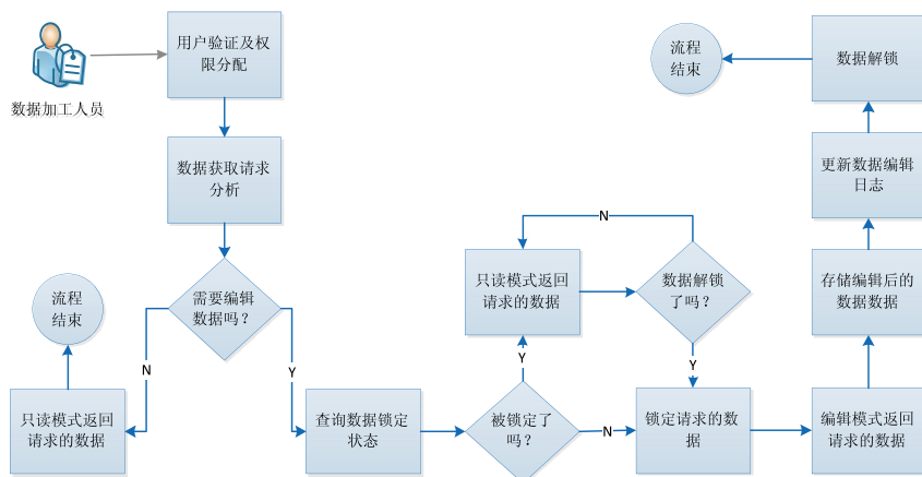
图2 workflow冲突解决机制
