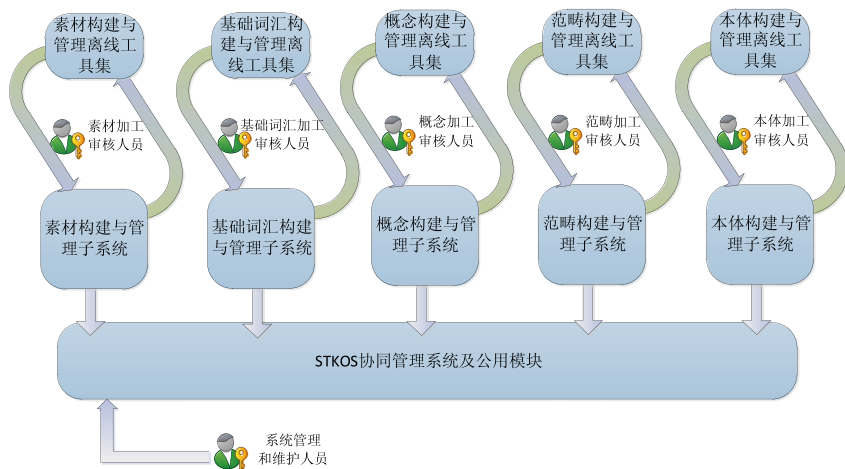
图1 分层循环工作流程
