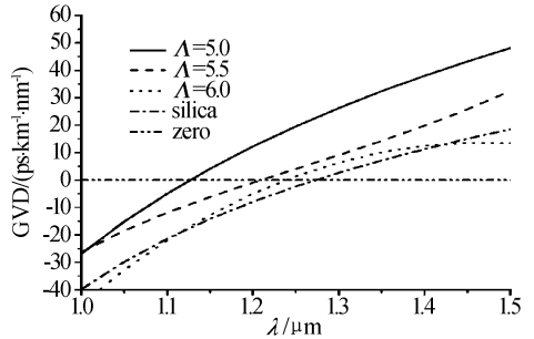
图 4 孔助光纤色散随空气孔位置的变化
