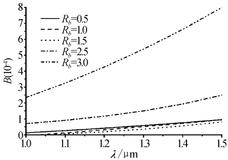
图5 改变 x 方向空气孔大小时双折射的变化情况
