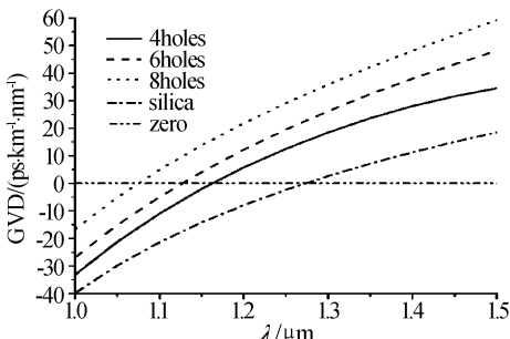
图 2 孔助光纤色散随空气孔数目的变化
