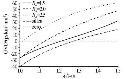
图 3 孔助光纤色散随空气孔大小的变化
