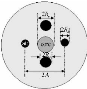
图 1 孔助光纤横截面结构及其参数示意图
