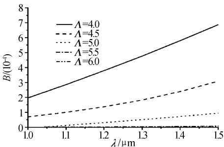
图6 改变空气孔位置时双折射的变化情况
