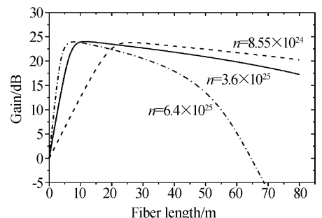
图 6 不同掺铒离子掺杂浓度下的增益与光纤长度的关系
