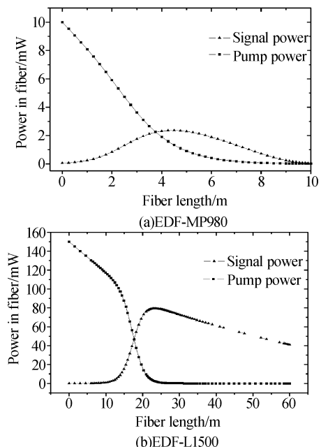
图 3 泵浦与最佳光纤长度的关系: \lambda_p = 980 nm, P_s^{in} = -10 dBm
