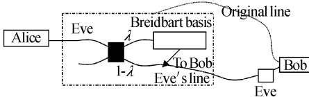
图 3 Eve 的窃听装置图
