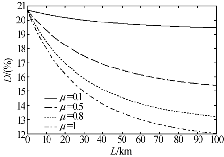
图 4 误码率与传输长度和平均光子数关系图
