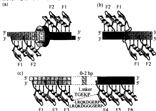
图3 多锌指串联以识别更长的DNA序列
