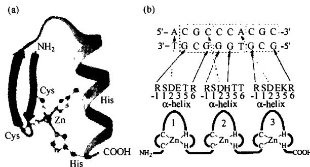
图 1 锌指单元的结构以及 C 2 H 2 型锌指 Zif268 与 DNA 的识别作用模式
