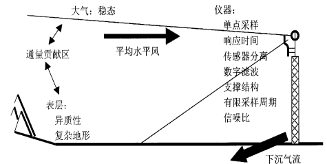
图 1 评价湍度相关系统通量测定结果有效性需考虑的主要过程及项目
