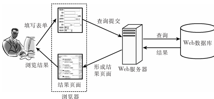
图 1 从 Web 数据库中获取数据的过程
