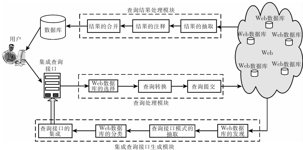
图 3 Deep Web 数据集成框架
