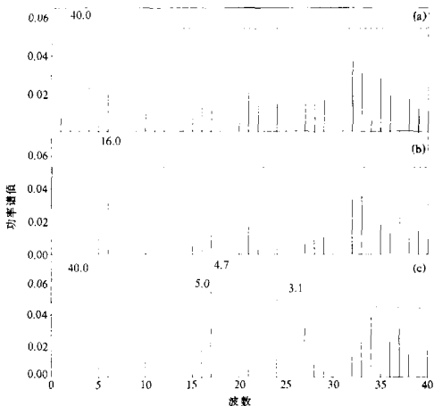
图 4 1880~1999 年副高 (a) 强度 (b) 西界 (c) 北界的功率谱 光滑实线为各自 95% 信度水平
