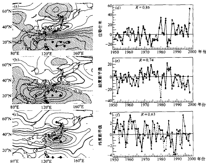
图1 1951~1998年(80°E~180°, 10~70°N)夏季国家气候中心500 hPa高度场与国家气候中心副高(a)强度、(b)西界、(c)北界指数的相关图和利用国家气候中心给出的高度场计算的副高指数与国家气候中心的副高指数距平值(d)强度、(e)西界、(f)北界 阴影表示相关系数绝对值大于0.3 ---▲---为计算的副高指数距平, —■—为国家气候中心给出的副高指数距平
