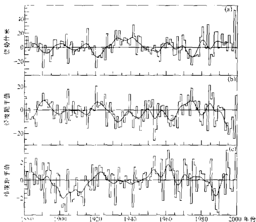
图3 1880~1999年副高(a)强度、(b)西界、(c)北界距平 图中光滑曲线为9年低通滤波值
