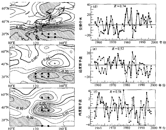
图2 1958~1997年(80°E~180°, 10~70°N)夏季NCEP 500 hPa高度场与国家气候中心副高 (a)强度、(b)西界位置、(c)北界位置的相关图和利用NCEP高度场计算的副高指数距平 与国家气候中心的副高指数距平(d)强度、(e)西界位置、(f)北界位置 图注同图1
