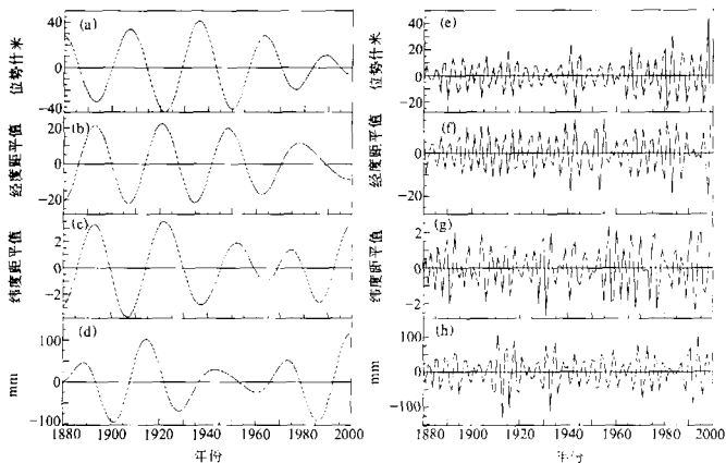
图8 1880~1999年副高(a)强度、(b)西界、(c)北界、(d)降水的28年周期部分和1880~1999年副高(e)强度、(f)西界、(g)北界、(h)降水的3.5年周期部分
