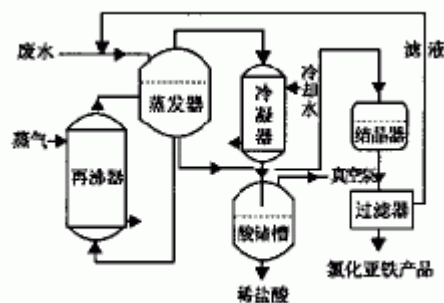
图1 高酸高铁废水回收稀盐酸与氯化亚铁的工艺流程图
