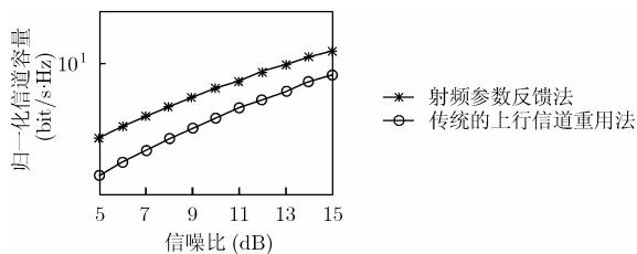
图3 发射天线为4接收天线为2时采用不同方法获取CSIT的信道容量比较
