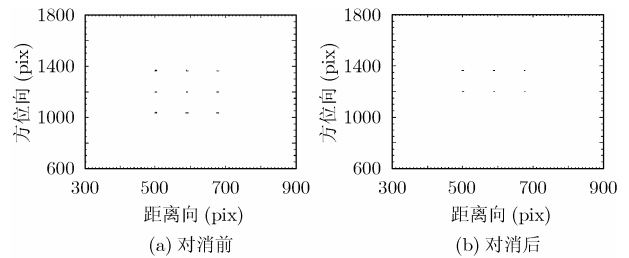
图 5 沿航迹干涉检测法仿真结果
