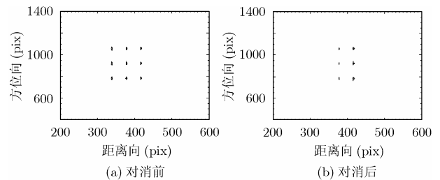
图 6 跨航迹干涉检测法仿真结果
