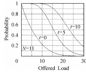
图 6 t 对分组成功传输概率和负载关系的影响 Fig.6 Probability P vs. G for different t
