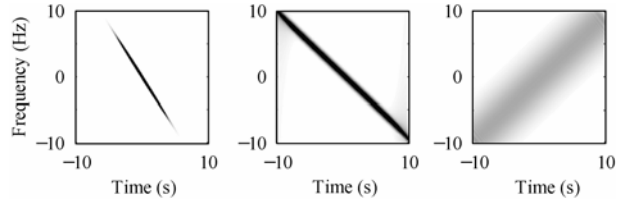
图 1 窗函数的 WVD 和两个 LFM 信号的谱图
