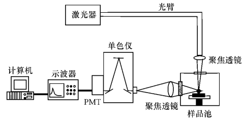
图1 LIBS实验装置图
