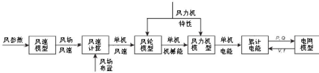
图 6 变速风力机集总模型结构
