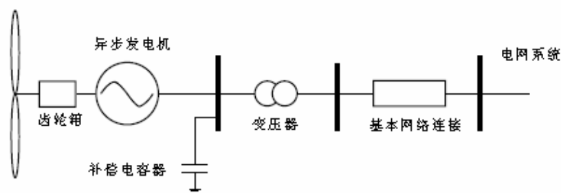
图 1 恒速风力机系统示意图
