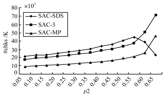
(b) 检查次数 (b) Check numbers
