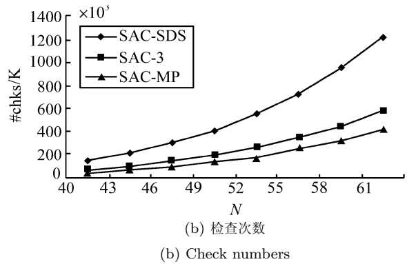
图 3 N 皇后问题 Fig.3 N queens problems
