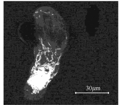
图 3 黑松的花粉粒经过离子注入后,其花粉管顶端的微丝网络丧失
