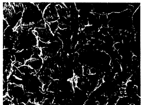
图 3 CLAM 钢 -196\text{ }^{\circ}\text{C} 冲击断口形貌
