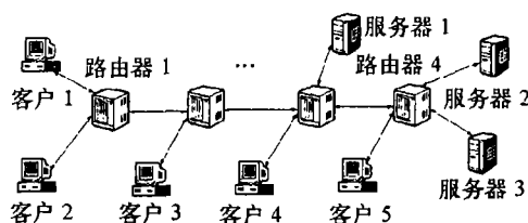
图 7 多链路网络仿真模型
