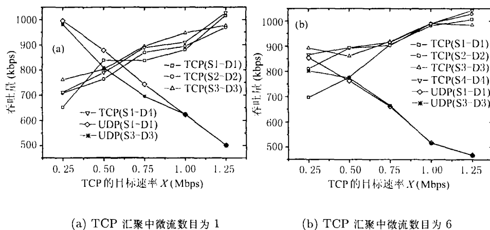
图 5 直接拥塞控制机制仿真结果
