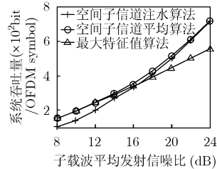
图 3 几种算法性能比较
