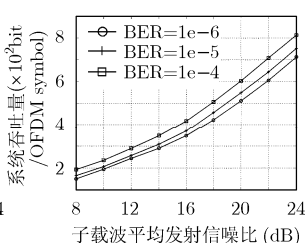
图 5 不同误比特率约束下的系统吞吐量
