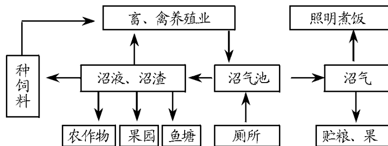
图1 北方四位一体模式
