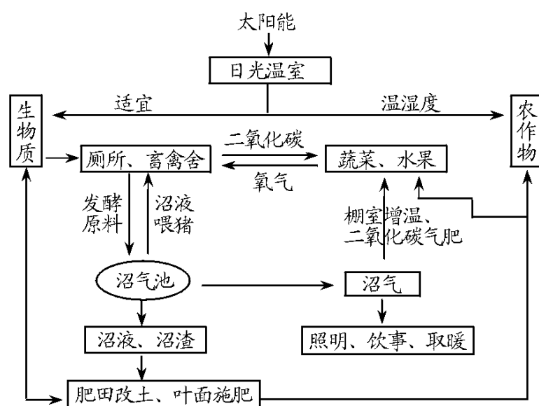
图1 北方四位一体模式
