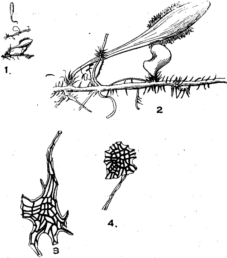
圖1 小伏石蕨, 新种
