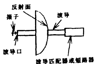
图 1 波导激励振子馈电的抛物面天线
