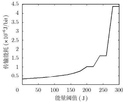
图 3 在误码率为 0.001 时,传输 1bit 的传输能耗上限受能量阈值的影响曲线
