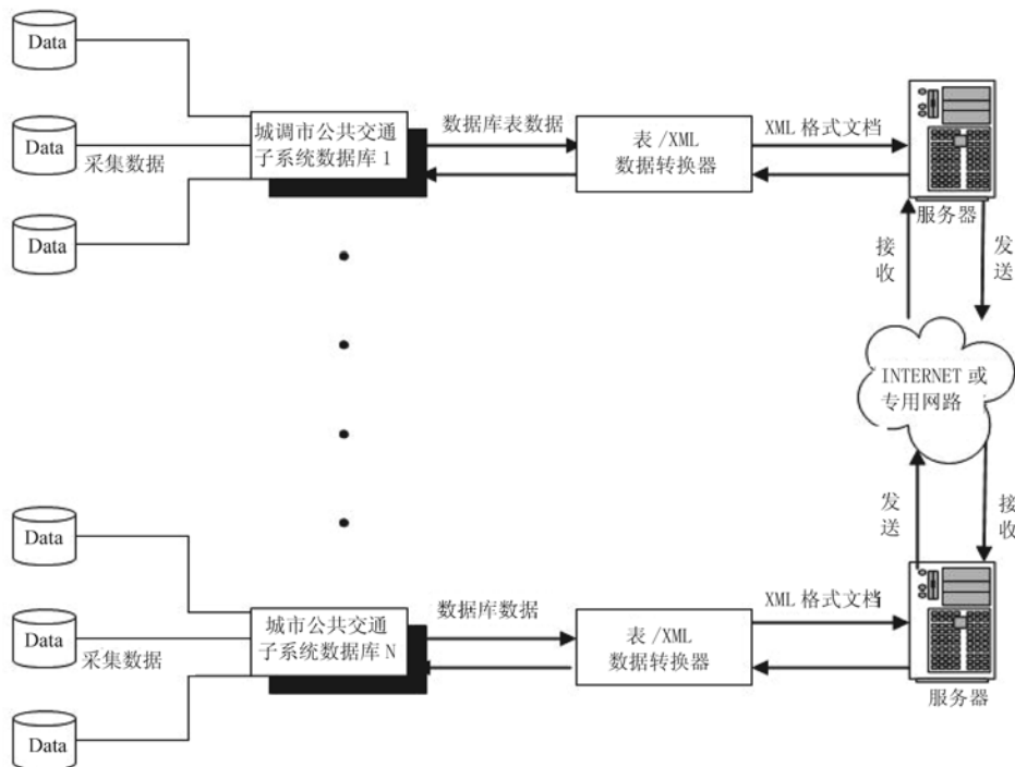
图3 城市公共交通信息数据交换系统体系结构
