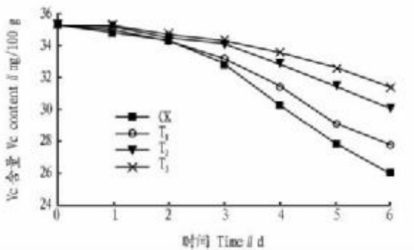
图5 草莓贮藏过程中 Vc 含量的变化
