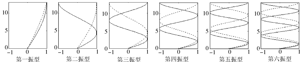
图5 悬挂结构挂于顶层时的前六阶振型图
