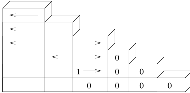
FIG. 4. \mu = (r)
