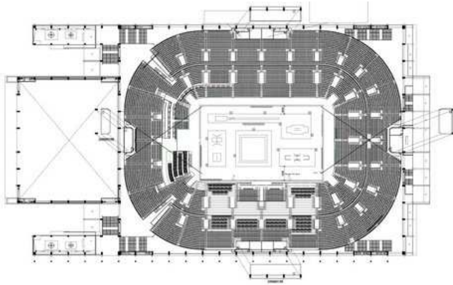
五层平面
