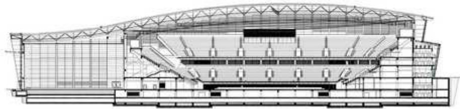
剖面
