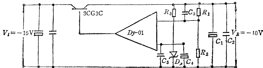
图 3 基准电源原理图
