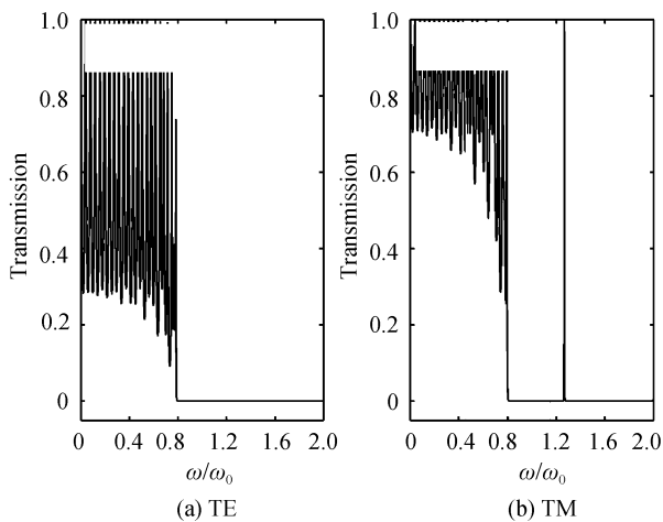
图 8 磁性材料无色散情况下电磁波 45^\circ 入射 TM 偏振滤波器时各偏振波的透射谱
