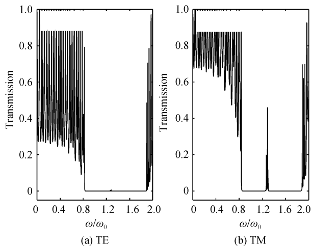
图 9 磁性材料低色散情况下电磁波 45^\circ 入射 TM 偏振滤波器时各偏振波的透射谱
