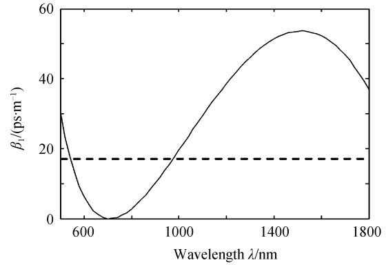
图 2 一阶色散系数随波长的变化
