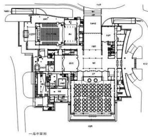
一层平面图
