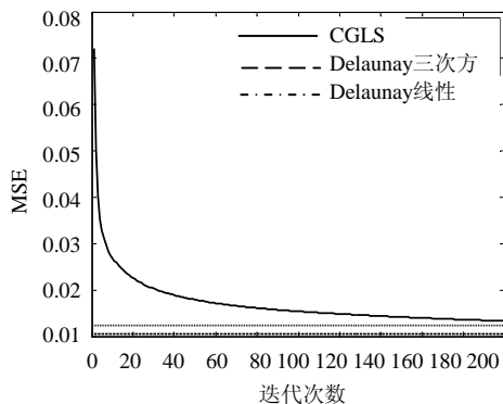
图1 重建均方误差比较
